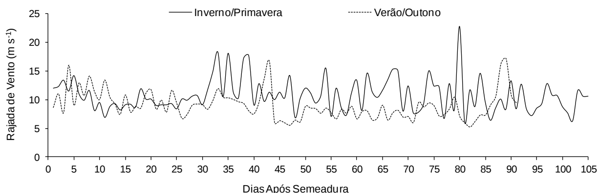
Figura 8. Máxima velocidade diária de vento (rajada de vento em \text{m s}^{-1} ) durante o ciclo da cultura do milho doce em duas épocas de cultivo. Chapadão do Sul - MS, UFMS-CPCS, 2012-2013.
