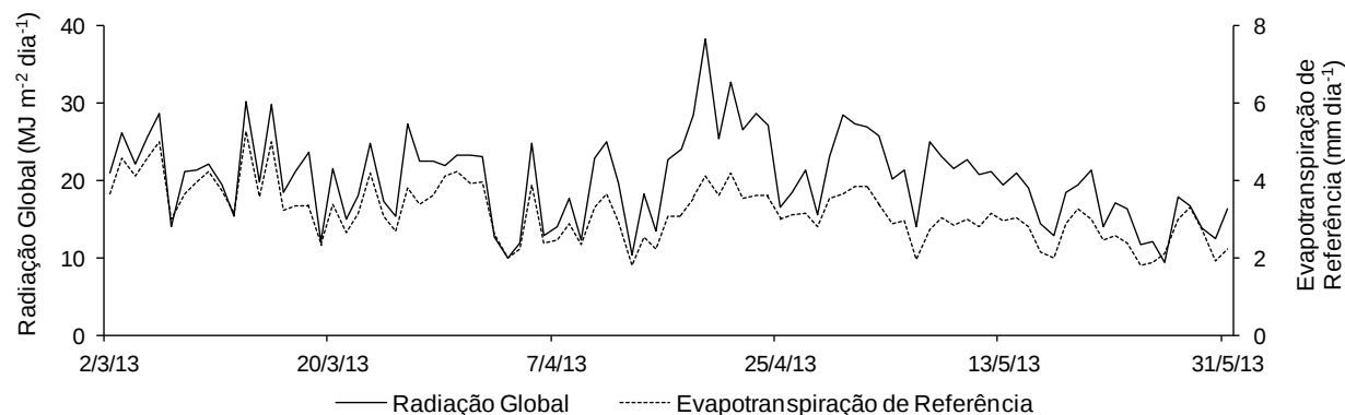
Figura 5. Variação diária da radiação solar global ( \text{MJ m}^{-2} \text{ dia}^{-1} ) e evapotranspiração de referência ( \text{mm dia}^{-1} ), nas épocas de cultivo: (A) Inverno/Primavera e (B) Verão/Outono. Chapadão do Sul - MS, UFMS-CPCS, 2012-2013.
