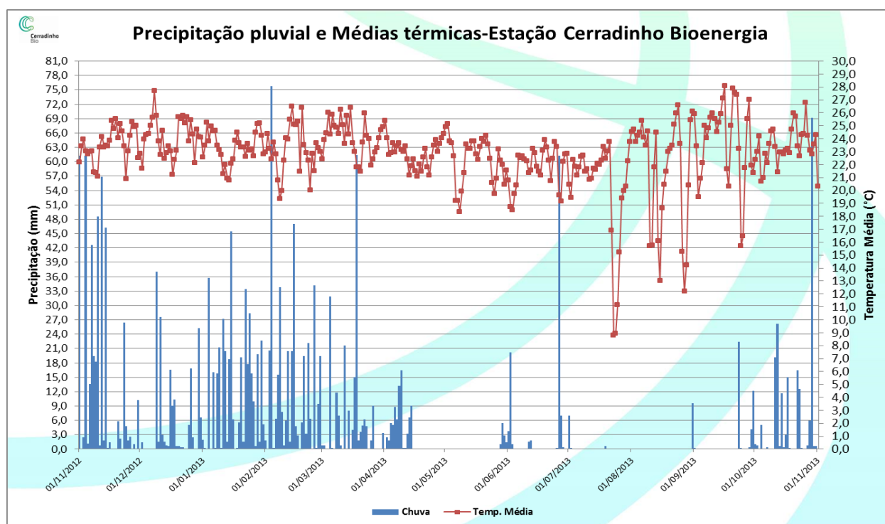
Figura 2: Precipitação pluvial e médias térmicas, obtidas na área experimental, durante o período de novembro de 2012 a novembro de 2013.
