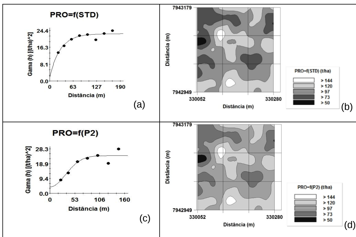
Figura 7. Semivariogramas cruzados e mapas de cokrigagem da PRO em função do STD, PRO em função do P2 de um Latossolo Vermelho-Amarelo distrófico de Chapadão do Céu, GO.
