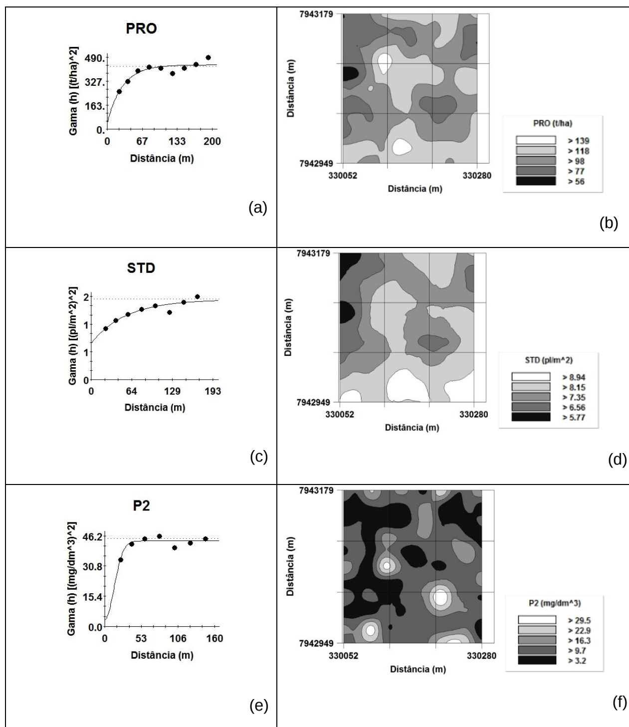
Figura 8. Semivariogramas simples e mapas de krigagem da PRO, do STD e do P2 de um Latossolo Vermelho-Amarelo distrófico de Chapadão do Céu, GO.
